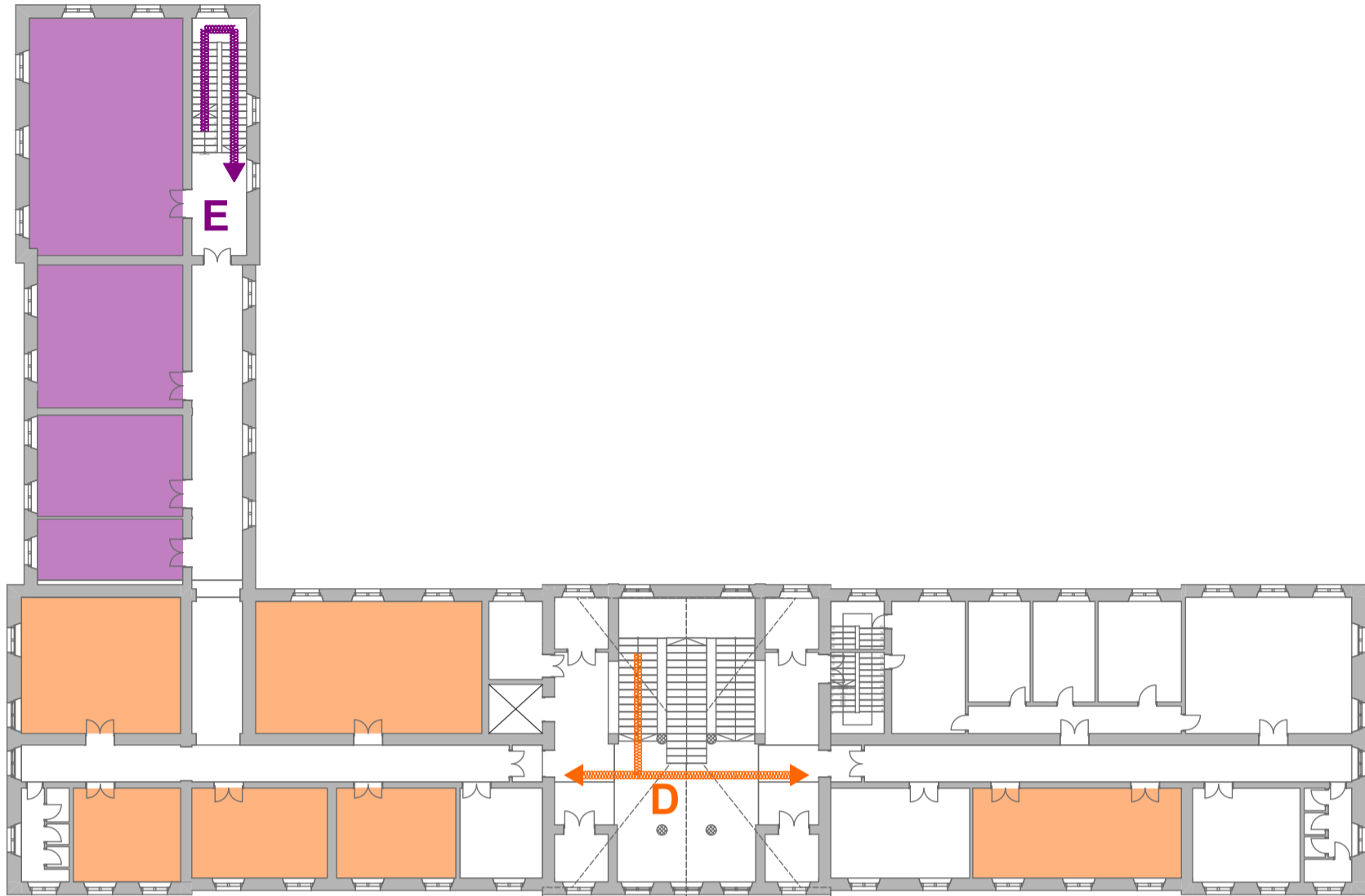
PIANO PRIMO
